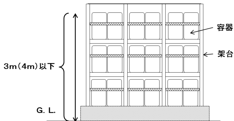
第3-6-4図 容器を積み上げる場合の例
