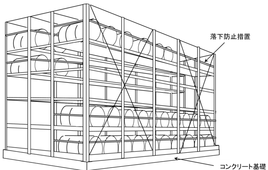
第 3-5-6 図 架台の構造の例
