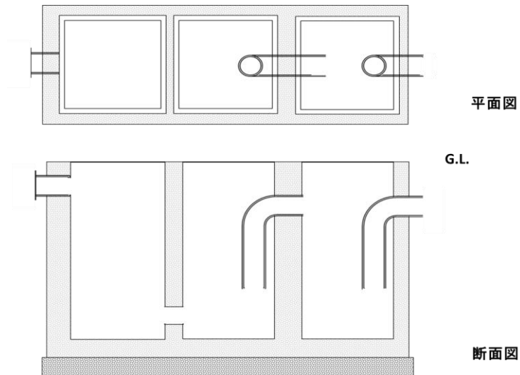
第 3-5-5 図 ためますを含めた油分離槽の例
