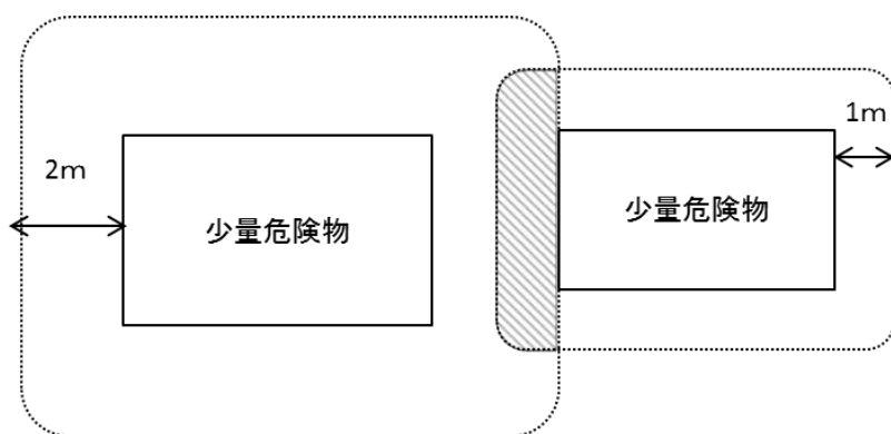
第3-5-2図 複数の少量危険物施設を隣接して設置する場合の例
