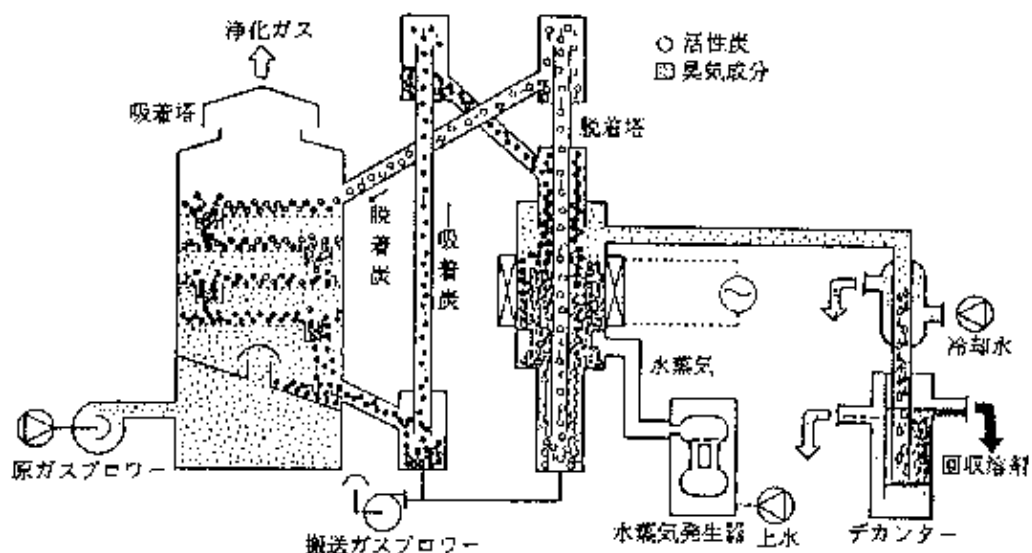
第 1 - 6 - 3 図 活性炭の流動方式
