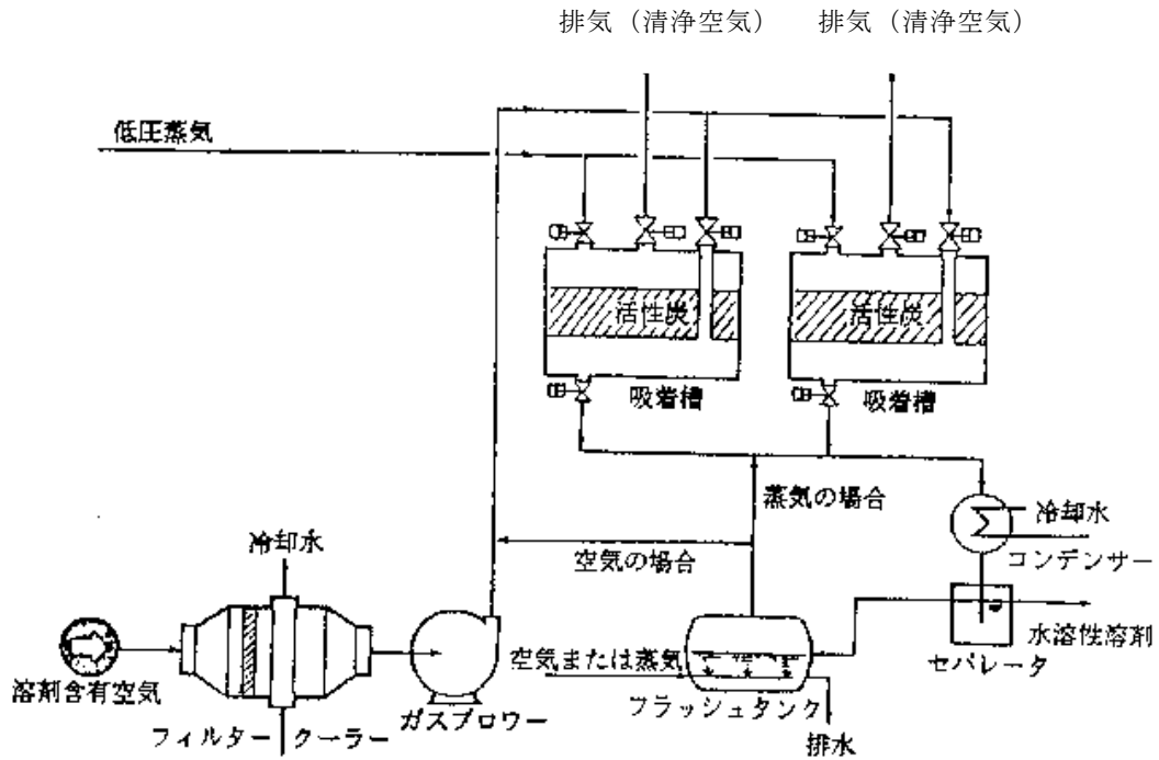
第 1 - 6 - 1 図 活性炭の固定層方式
