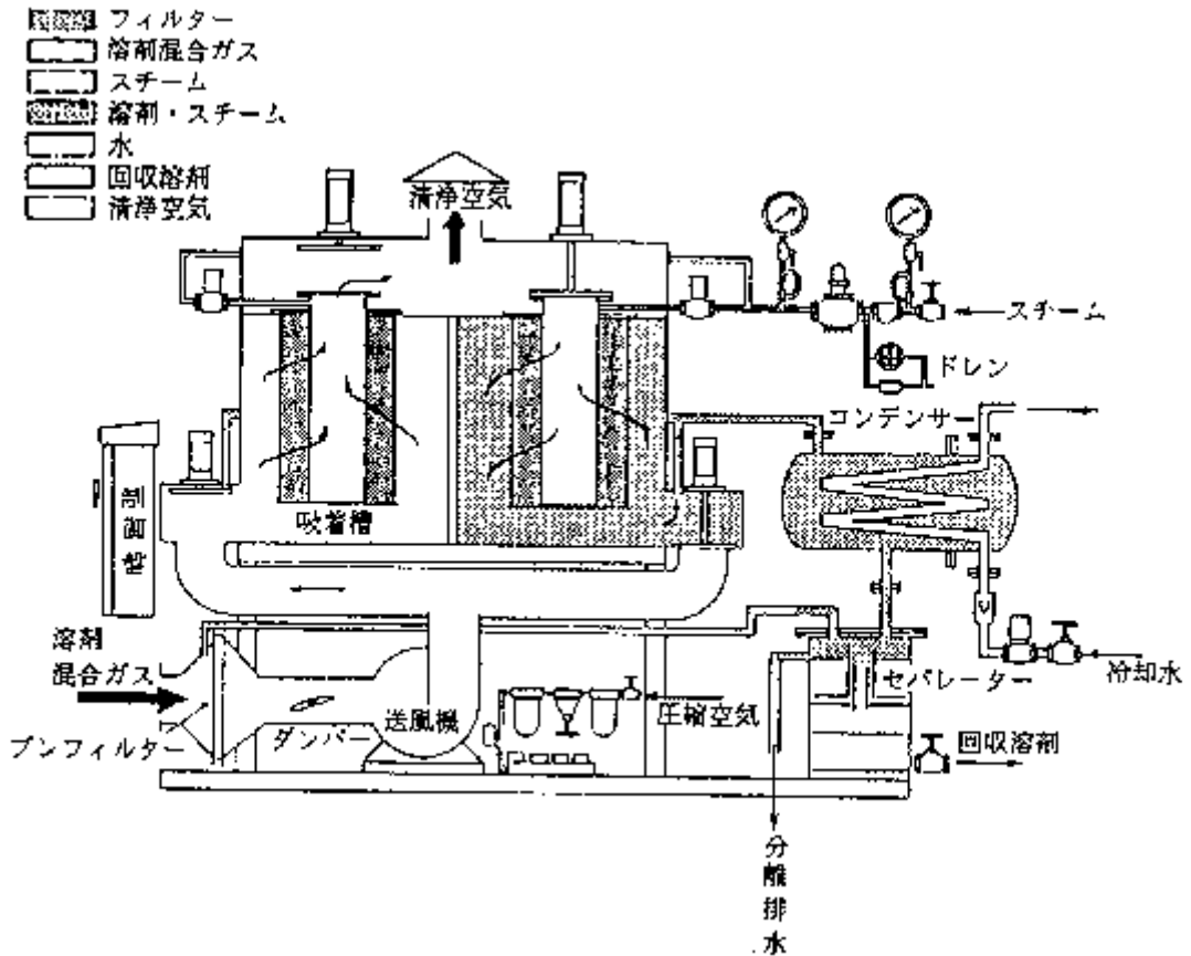
第 1 - 6 - 2 図 活性炭のフィルター方式
