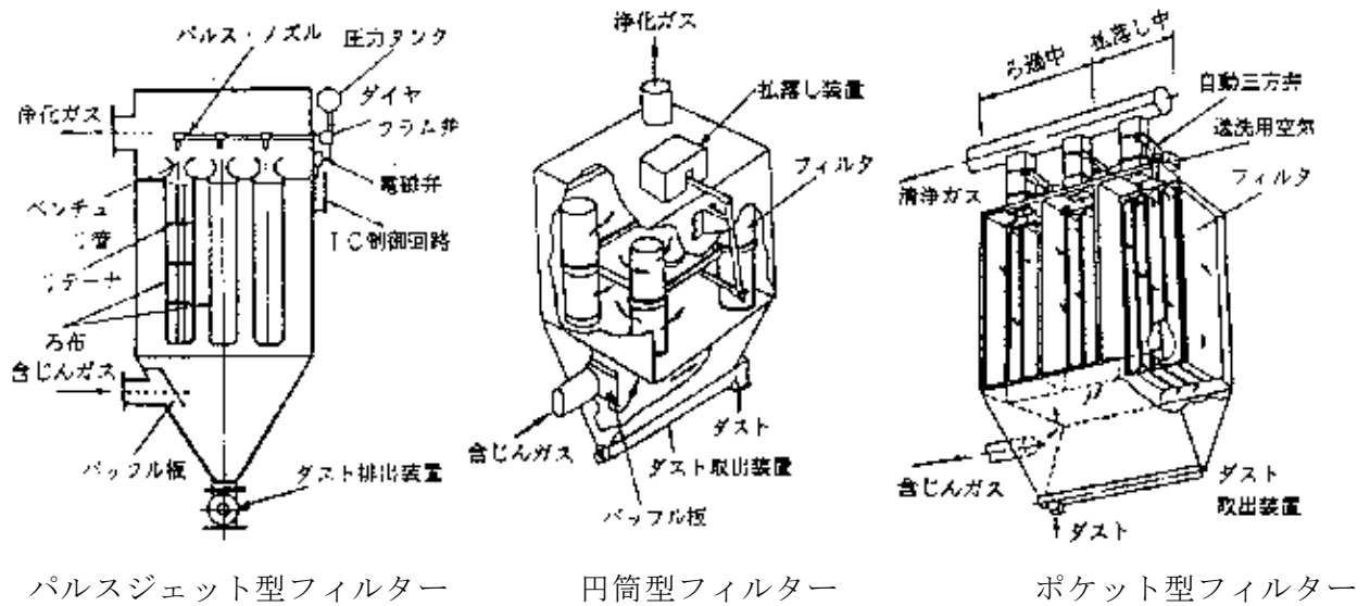
第 1 - 6 - 4 図 バグフィルターの構造例
