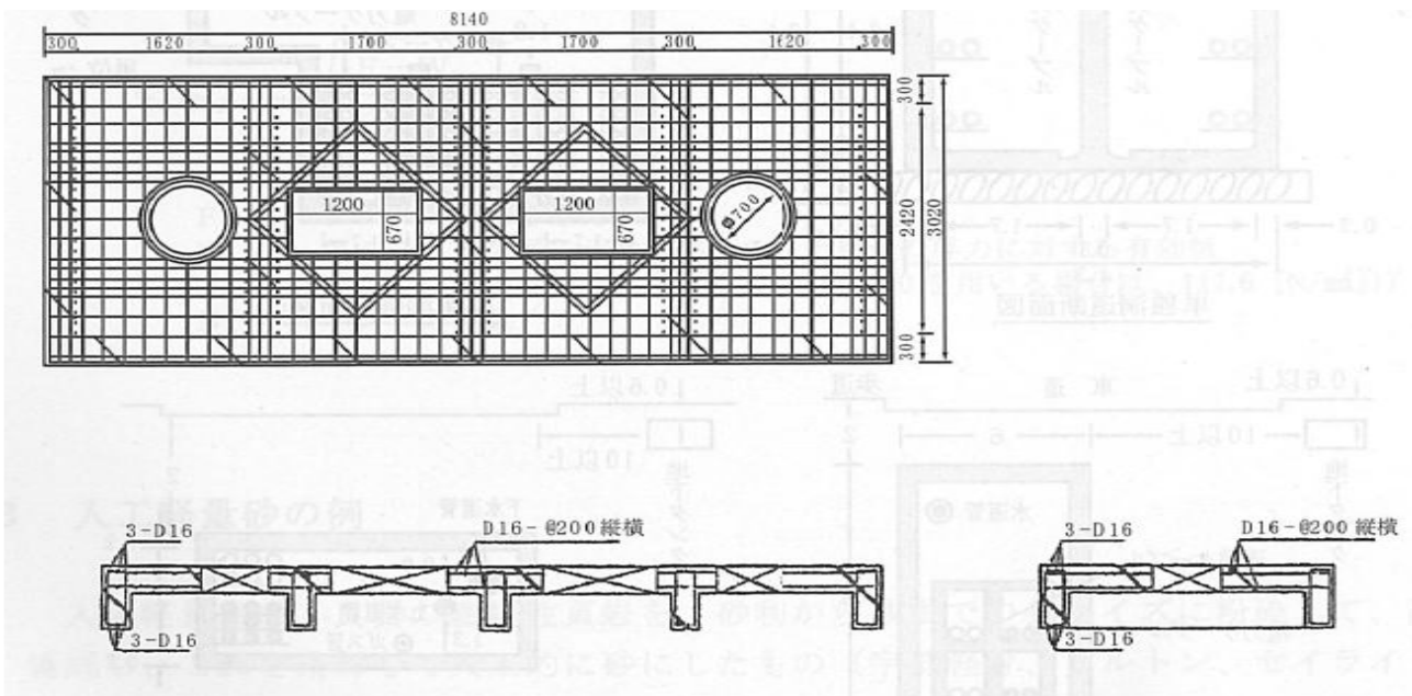
第5-7-2図 コンクリート被覆タンク配筋図 [30k \phi 、中仕切15:15 (直径2.4m)]
