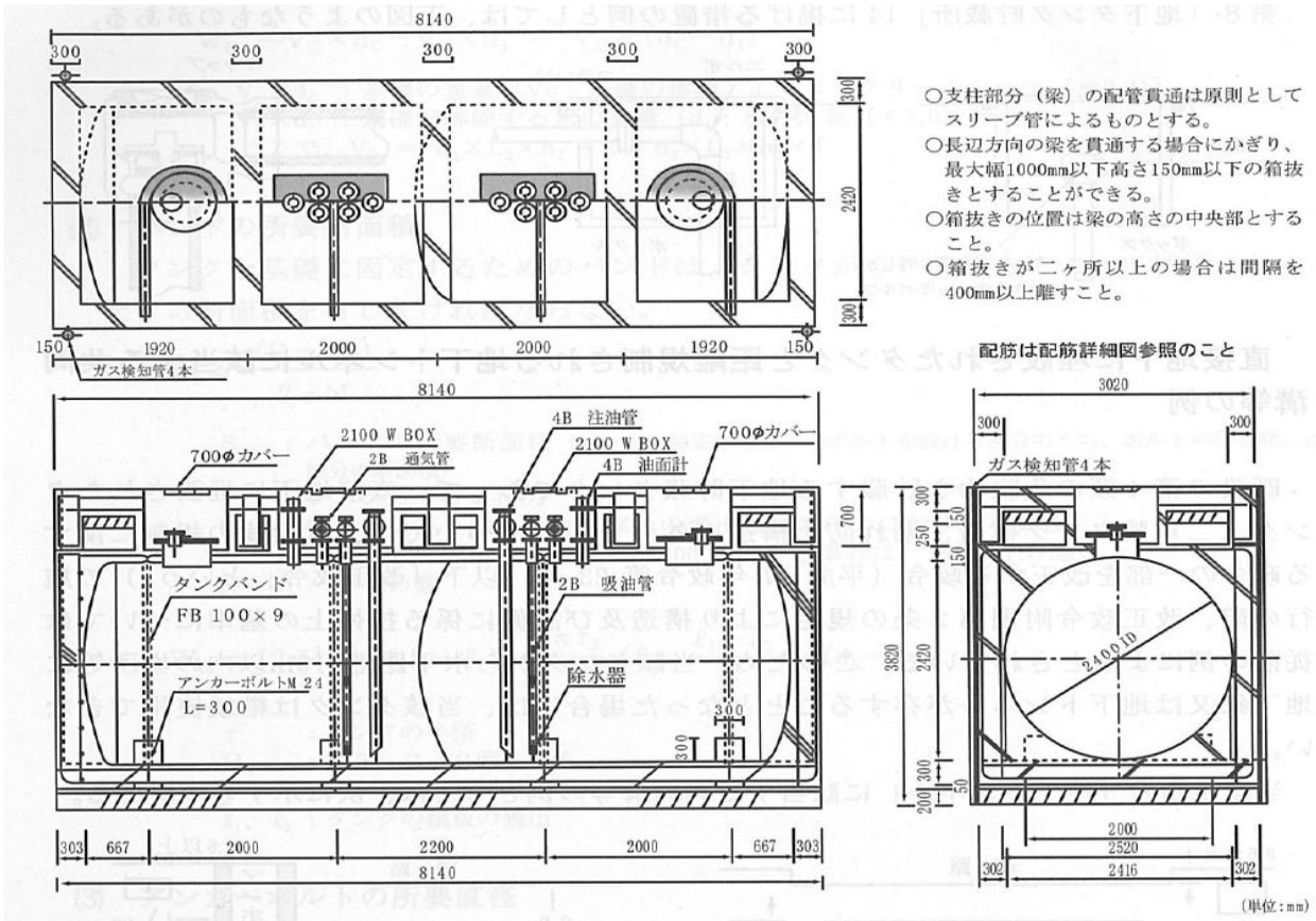
第5-7-1図 コンクリート被覆タンク埋設図 [30k \phi 、中仕切15:15 (直径2.4m)]
